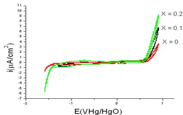
Figure 4 . Voltamogrammes relatifs à l'oxyde \text{Ca}_{1-x}\text{Sr}_x\text{MnO}_3 ( x = 0, 0.1, 0.2 )
