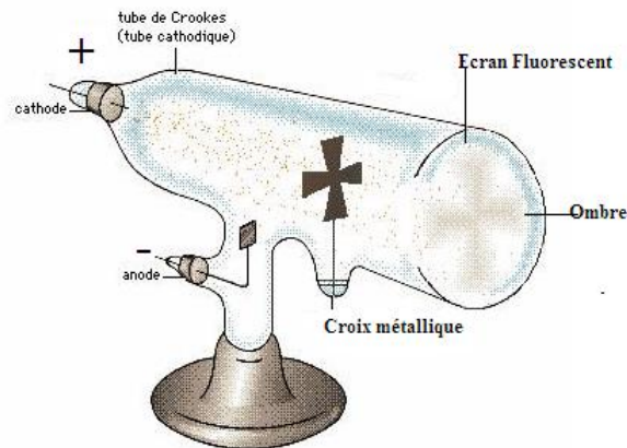
Schéma d'un tube de Crookes.
