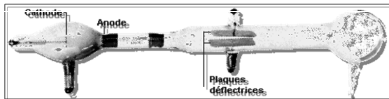
Schéma d'un tube de Crookes modifié par J.J. Thomson.
