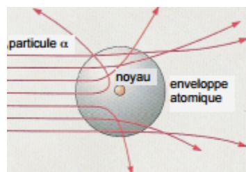
Modèle atomique de Rutherford
