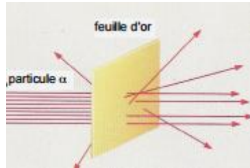
Expérience de diffusion de Rutherford
