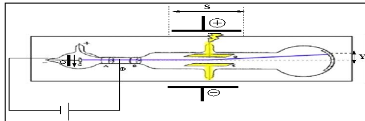
Expérience de J.J. Thomson.
