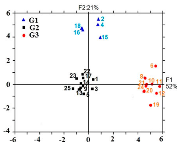
Fig. 10. Plots of PCA scores for F1 vs. F2.
