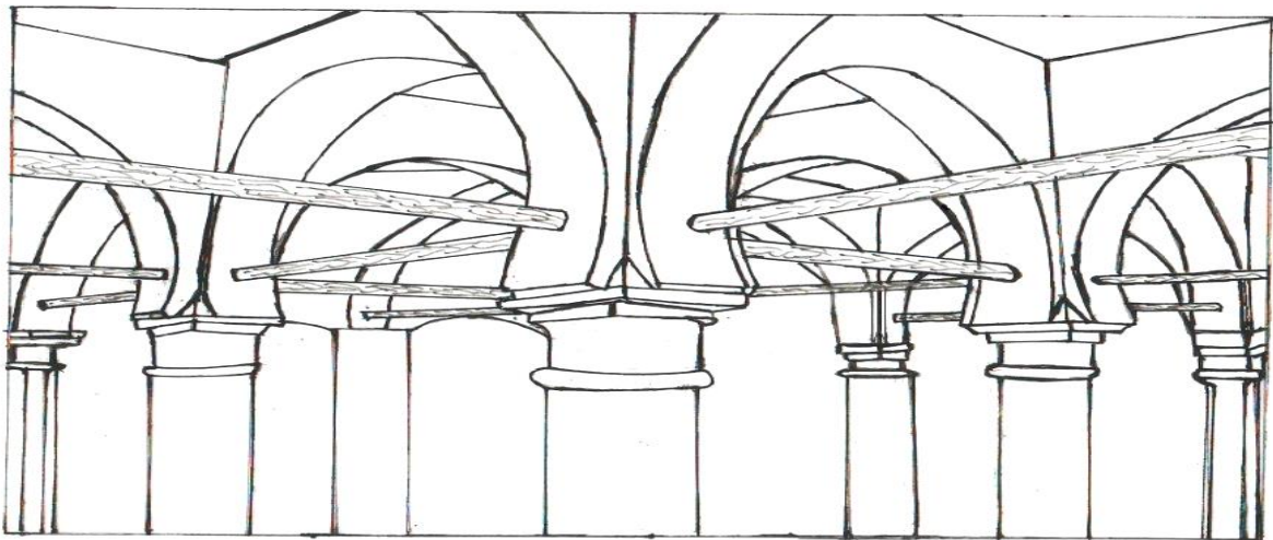
أعمدة بيت صلاة جامع بومرزوق الحاملة للعقود وأوتارها الخشبية
