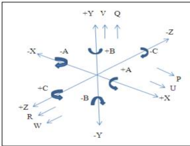
Figure. II.6 : Axes Primaires Et Axes Additionnels. [10]
