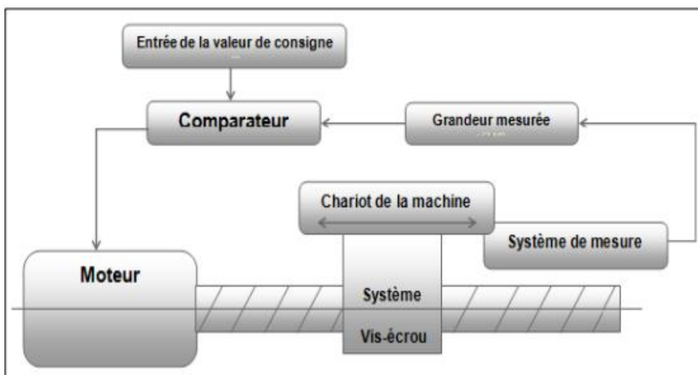
Figure II.4 : Commande en boucle fermée. [10]
