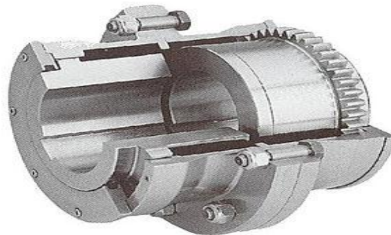
Figure. I.4 : Accouplement à engrenages. [3]
